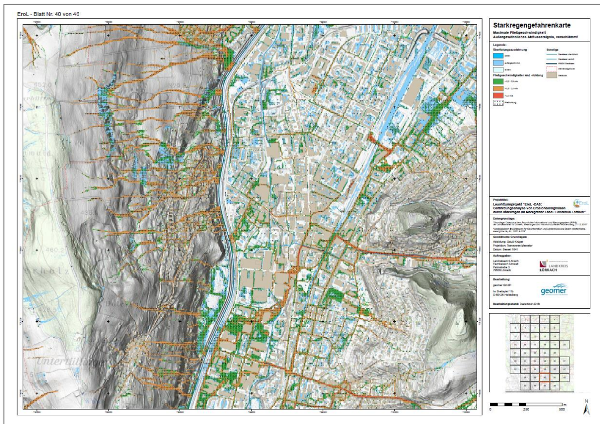
Abb. 37: Maximale Fließgeschwindigkeitskarte mit maximaler Ausdehnung der Überflutung des außergewöhnlichen Abflussereignisses im EroL Projektgebiet
