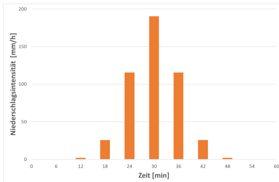
Abb. 24: Zeitlicher Verlauf der mittelbetonten mittleren KOSTRA-Niederschlagsganglinien im 6-Minuten-Intervall im EroL-Einzugsgebiet (30-jährliche Wiederkehrzeit (D60T30))
