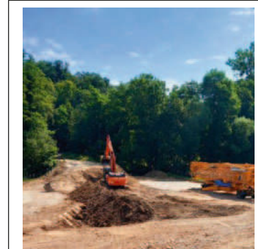
Wintersweiler, Regenüberlaufbecken
