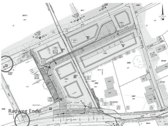
Lageplan Neubaugebiet Brühl, Egringen
