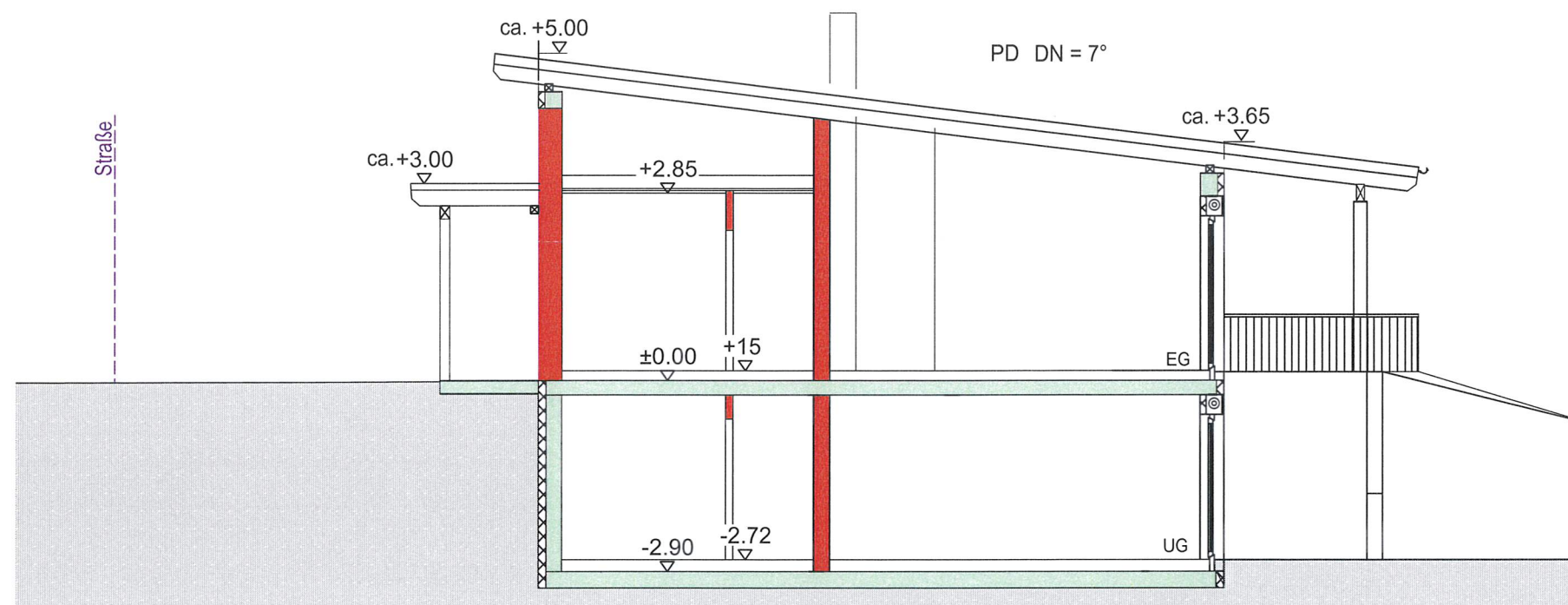
Schnitt A-A
